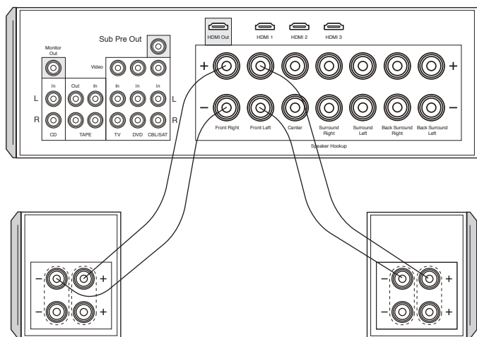
Рисунок 5 Стандартное подключение
