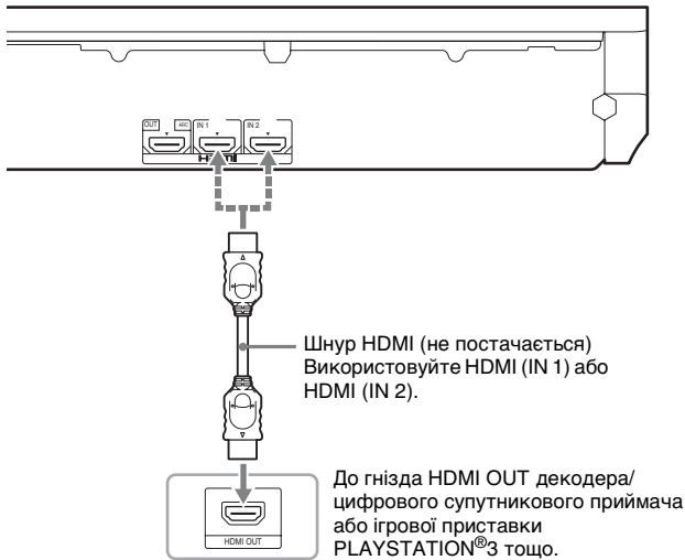
Задня панель пристрою
