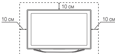
Встановлення на підставці.
