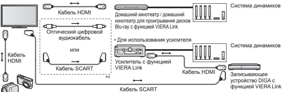
Видеокамера HD / фотокамера LUMIX с функцией VIERA Link
