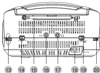
Общий вид задней панели
