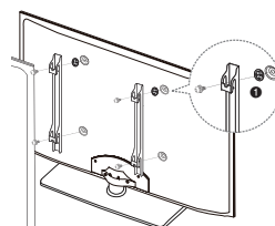
Вариант Б. Установка настенных креплений других производителей
