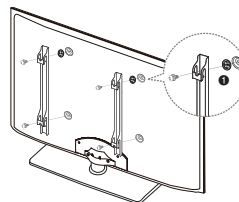
Спосіб Б. Встановлення настінного кріплення іншого виробника
