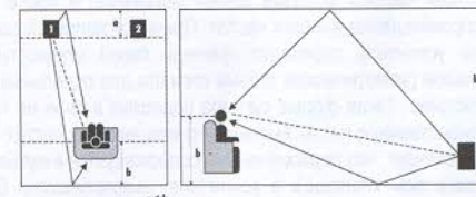
a ≠ b Несимметричное (лучшее) размещение
