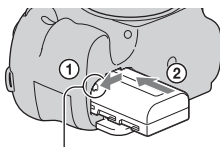
Vergrendelingshendel
