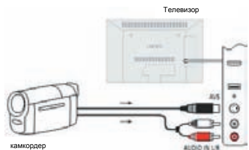
Пример подключения камкордера
