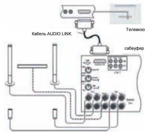
Подключение аудиосистемы Loewe (сабвуфер) к телевизору
