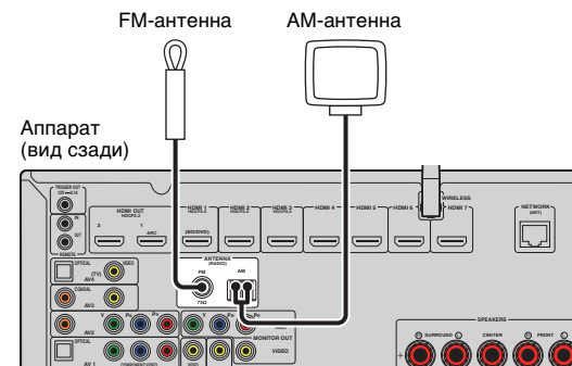
Сборка и подключение AM-антенны
