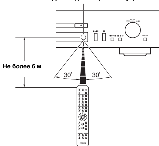
Датчик дистанционного управления
