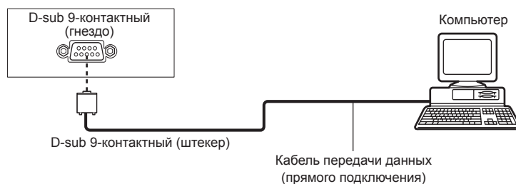
Подключение разъемов проектора
