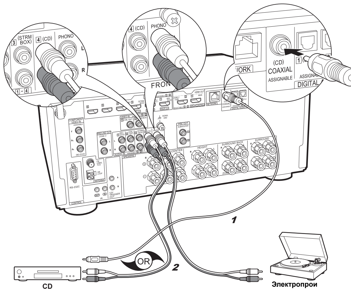
1 Цифровой коаксиальный кабель, 2 Аналоговый аудиокабель
