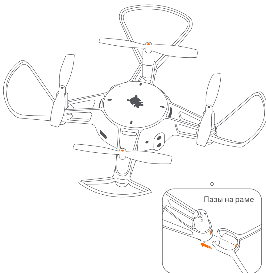
Совмещение выступов защитной рамы с пазами на раме
