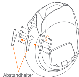
Abstandshalter
