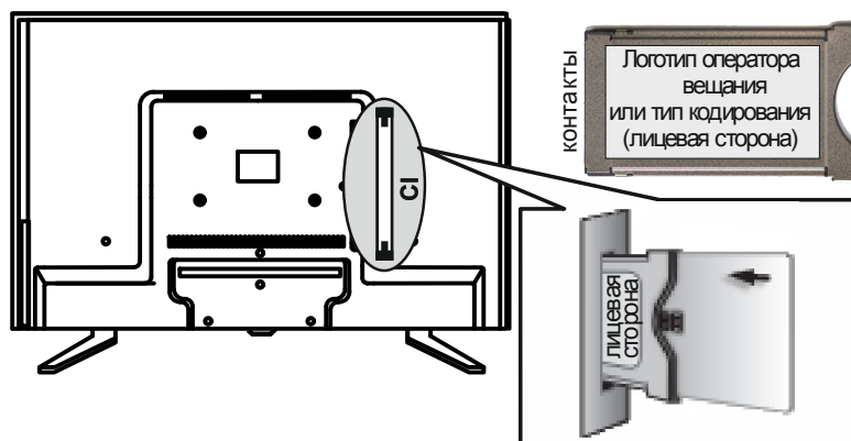
Рисунок 5 – Установка СА-модуля
