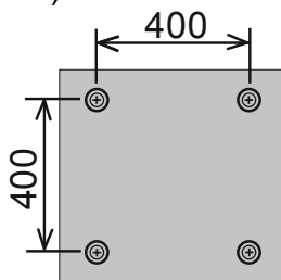
Рисунок 4 – Размеры для выбора настенного кронштейна
