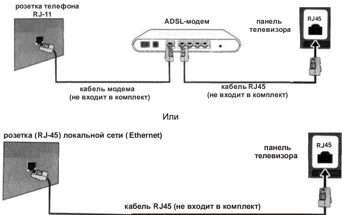
Рисунок 6 – Проводное подключение
