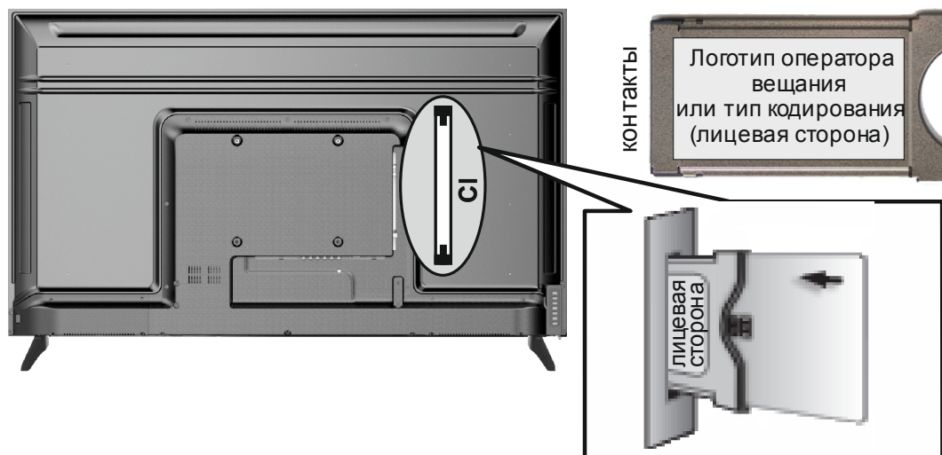
Рисунок 5 – Установка СА-модуля
