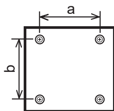
Рисунок 6 – Размеры для выбора настенного кронштейна
