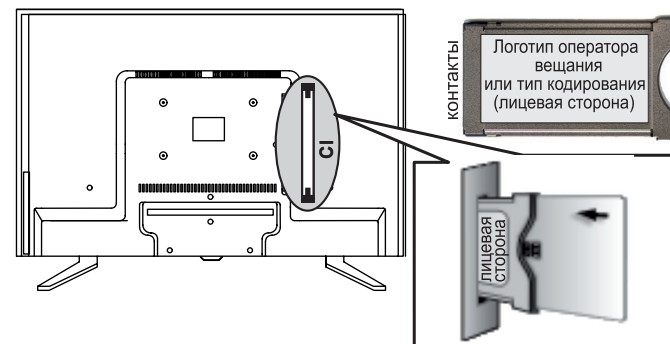
Рисунок 7 – Установка СА-модуля
