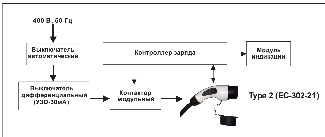
Рисунок 6 – Структурная схема станции EC-302-21
