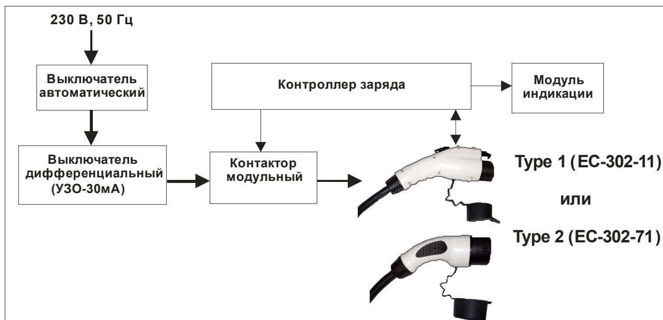
Рисунок 5 – Структурная схема станций EC-302-11, EC-302-71
