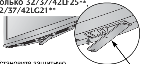
защитная крышка
