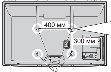
Отверстия для крепления настенного кронштейна
