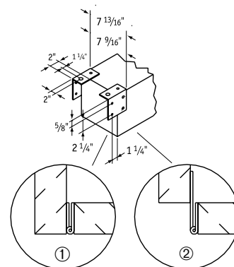
Способ установки экрана: 1 стандартной и 2 выносной конструкции
