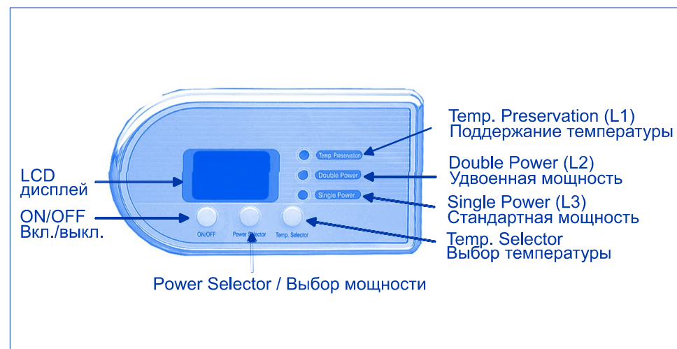
Рис. 4. Электронная панель управления (вариант 1)
