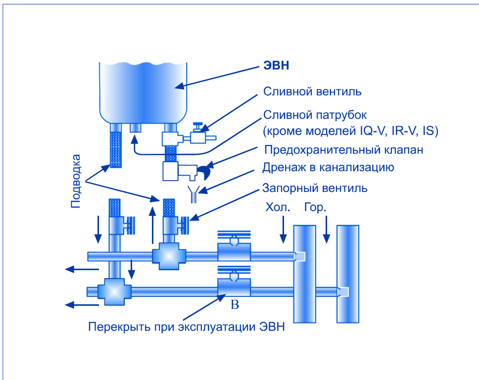
Рис 1. Схема подключения ЭВН к водопроводу
