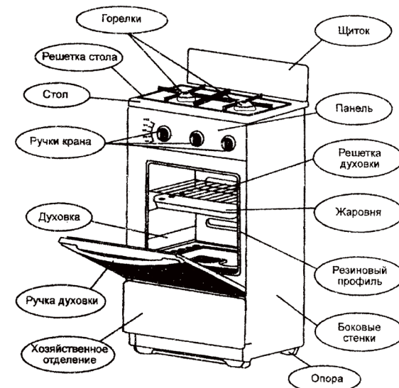
Рис. 2 Газовая плита с 2 горелками
