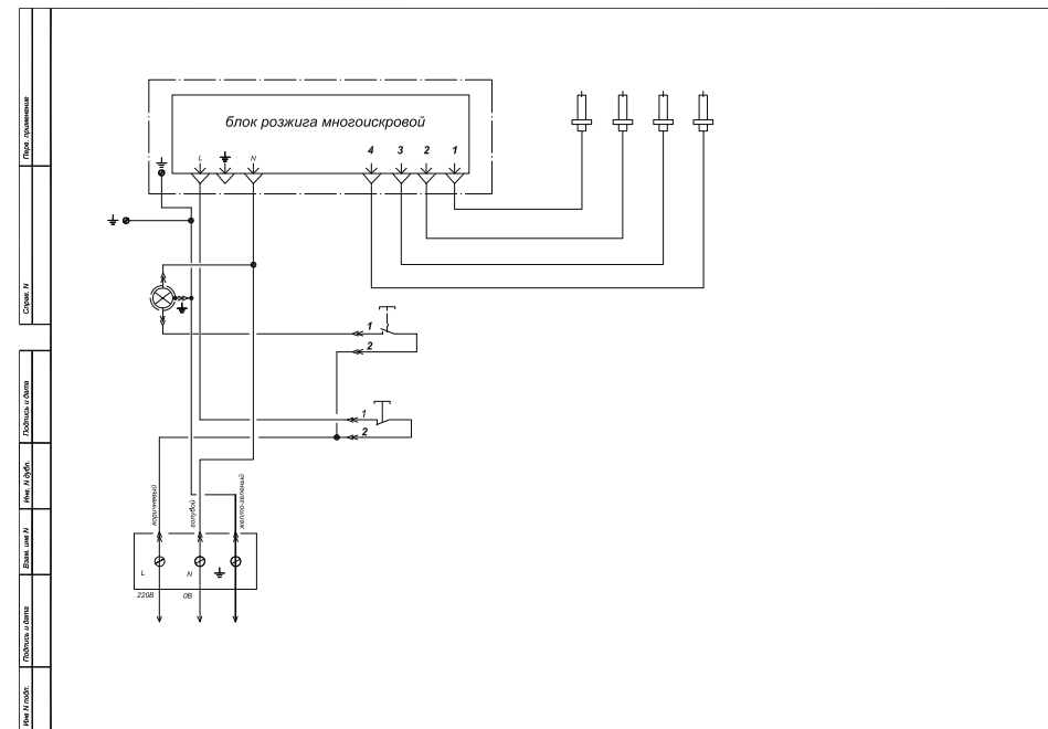
Рис. 8. Схема электрическая принципиальная
