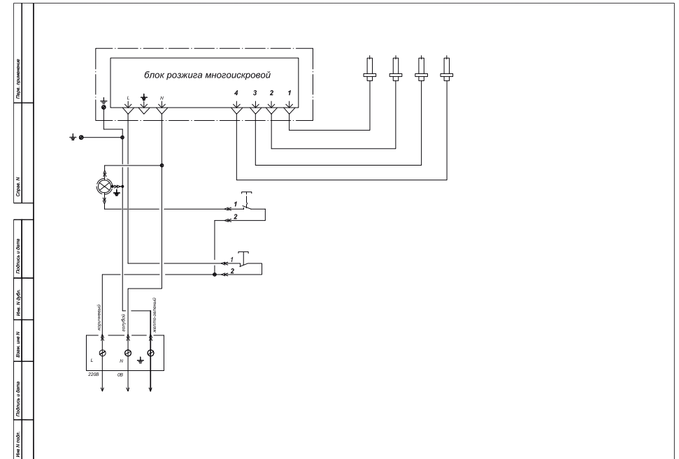
Рис. 8. Схема электрическая принципиальная
