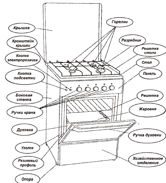
Рис. 1 Газовая плита с 4 горелками
