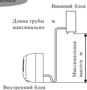
Схема установки
