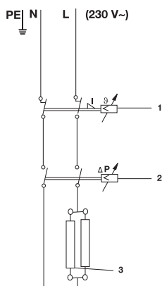
Рис. 6. NP Aquatronic
