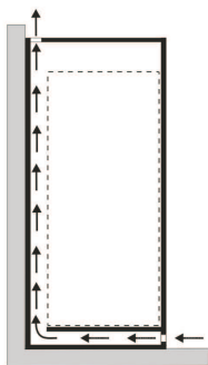
Рисунок Б.7 - Схема циркуляции воздуха вокруг холодильного прибора Рисунок Б.7 - Схема циркуляції повітря навколо холодильного приладу Şəkil B. 7. - Soyuducu cihazın ətrafında havanın dövriyyə sxemi Сурет Б.7 - Тоңазытқыш прибор айналасындағы ауа айналысының схемасы Figura B.7 - Schema de circulație a aerului în jurul instalației frigorifice B.7-rasm: : Sovutish uskunasing atrofigda havo aylanish chizmasi
