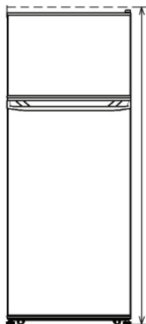
Рисунок Б.8 - Габаритное пространство - рабочие габаритные размеры Рисунок Б.8 - Габаритний простір Şəkil B. 8. - Qabarit space Сурет Б.8 - Пішндік кеңістік Figura B.8 - Dimensiuni de spațiu B.8-rasm: Габарит бұшлик
