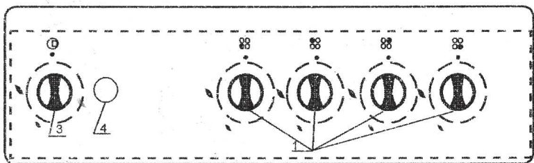
Панель плиты с терморегулятором и устройством предохранительным горелки духовки
