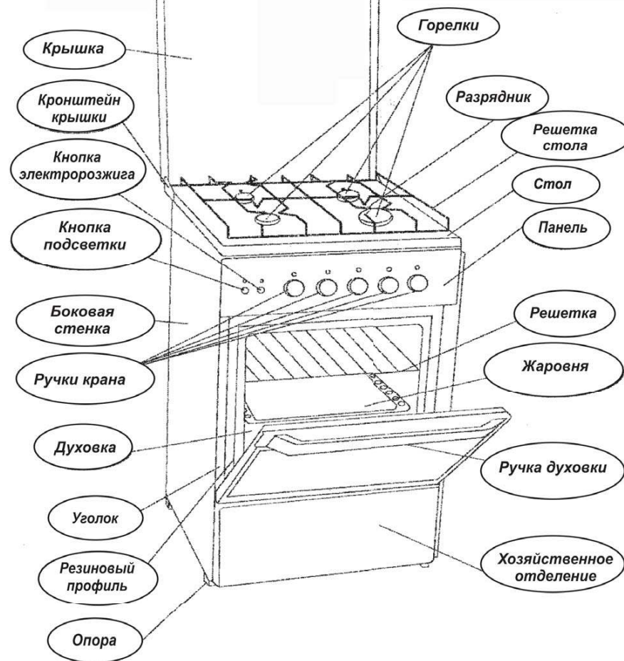
Рис. 1 Устройство плиты
