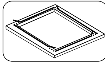
Наклеивание уплотнения на столешницу вдоль краев вырезанного отверстия
