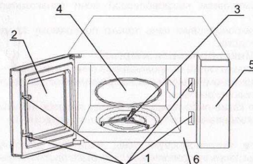
1 - Система замков двери, 2 - Дверь, 3 - Роликовая подставка, 4 - Стекланный поднос, 5 - Панель управления, 6 - Корпус
