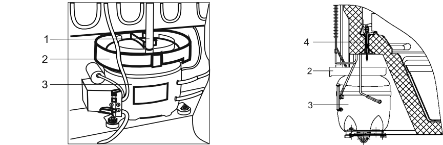
Рисунок Б.2 - Схема крепления упоров к крышке
