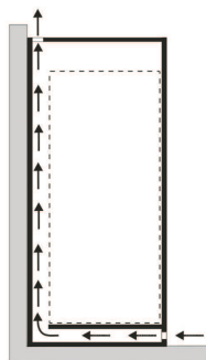
Рисунок Б.7 - Схема циркуляции воздуха вокруг холодильного прибора Рисунок Б.7 - Схема циркуляції повітря навколо холодильного приладу Şekil B. 7. - Soyuducu cihazın ətrafında havanın dövriyyə sxemi Сурет Б.7 - Тоңазытқыш прибор айналасындағы ауа айналысының схемасы Figura B.7 - Schema de circulație a aerului în jurul instalației frigorifice B.7-rasm: : Sovutish uskunasing atrofigda havo aylanish chizmasi
