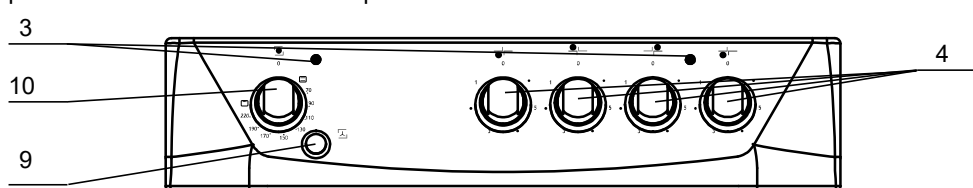
рис. 8. Панель плиты с совмещенной ручкой управления терморегулятора и переключателя мощности.
