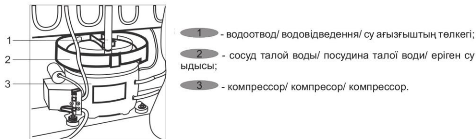
Рисунок Б.4 - Схема отвода талой воды из холодильной камеры Рисунок Б.4 - Схема відведення талої води з холодильної камери Б.4-сурет - Тоңазытқыш камерадаң еріген судың ағу сызбанұсқасы
