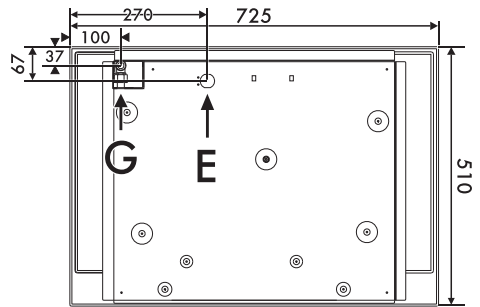
Вид снизу
