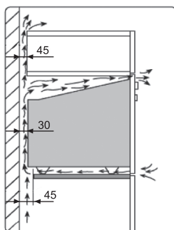
Рис. 4. Схема по встраиванию духового шкафа
