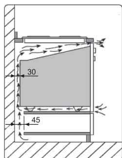
Рис. 4. Схема по встраиванию духового шкафа
