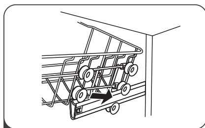
3 Насадите корзину на верхний (или нижний) ряд роликов.
