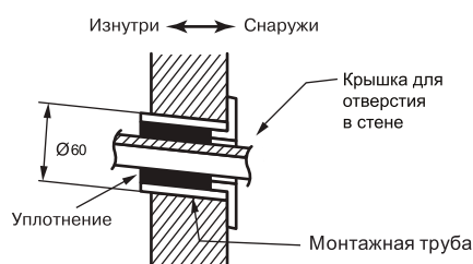
Монтажная труба
