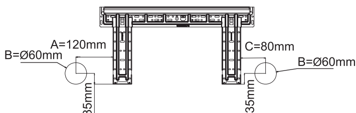
Монтажная труба
