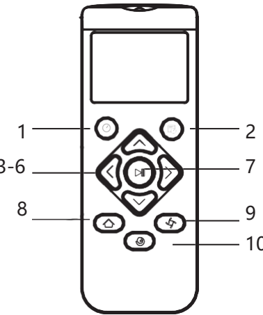
Пульт дистанционного управления с дисплеем (использование без приложения)
