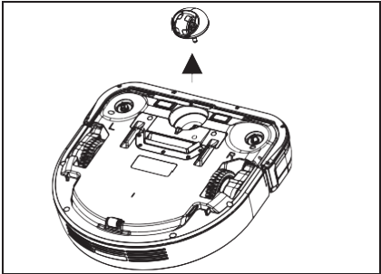
Направляющее колесо Потяните направляющее колесо вверх, затем очистите его.
