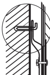
Вид сбоку
