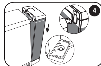
Réinsérer le réservoir au niveau des deux fentes et le repositionner vers le corps de la machine pour assurer sa complète fixation. Vérifier que le réservoir est correctement fixé.
