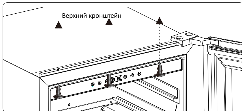
Винты (ST4.2*12мм)
