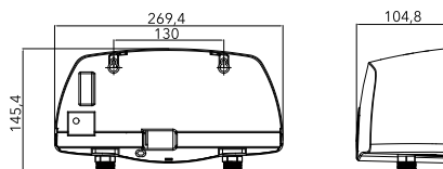
NP MINIFIX
