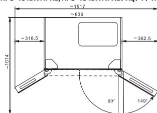
RFQ-490DX NFY / Xq / Xd / B / W / GY / GP / GB / GW / GR / GS / Ym
