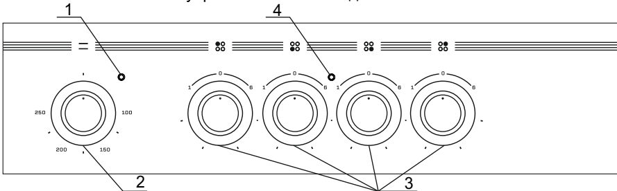
Панель управления плиты модели 506004.14эс
