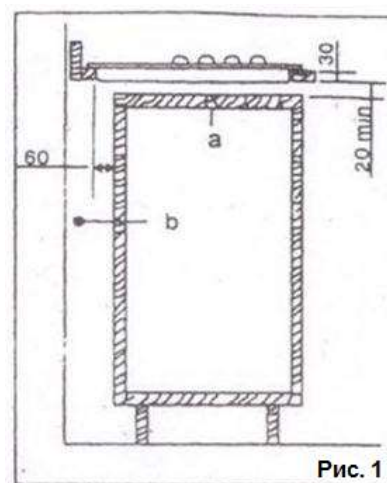
а съемная стенка b пространство для подключения
